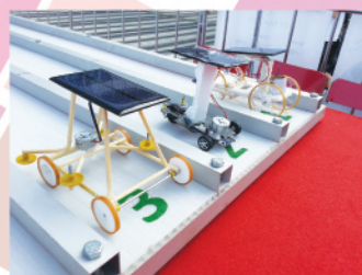
參賽太陽能車
